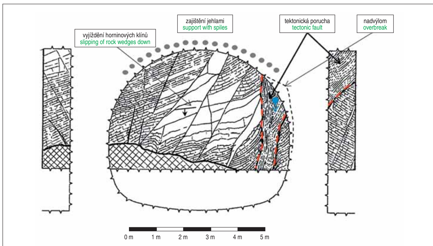
Obr. 5 Inženýrskogeologické sledování čela výrubu při ražbě přístupové chodby – nákres Fig. 5 Engineering geological monitoring of excavation face during excavation of the access gallery – drawing
