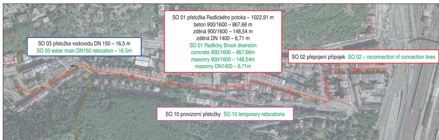
Obr. 6 Zákres přeložky potoka do ortofoto mapy
