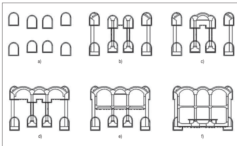
Obr. 3 Etapy výstavby stanice; (a) pomocné chodby/štolý, (b) výstavba pilot, sloupů a hlavních nosníků/průvlaků, (c) výstavba obloukové klenby střední lodi stanice, (d) výstavba obloukových kleneb bočních lodí stanice, (e) hloubení a výstavba horní etáže stanice, (f) hloubení a výstavba spodní etáže stanice
