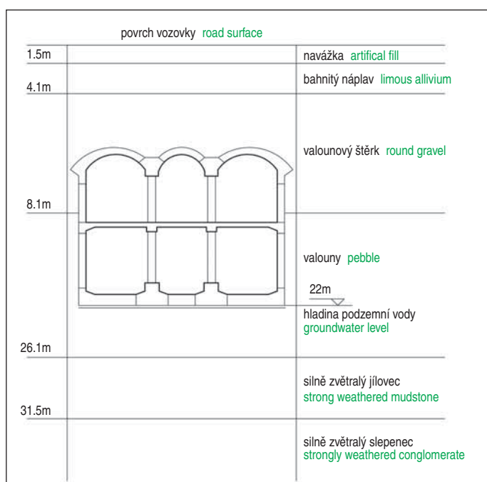
Obr. 1 Geologický profil prostředím stanice Qianmen Fig. 1 Geological profile of the Qianmen station environment
