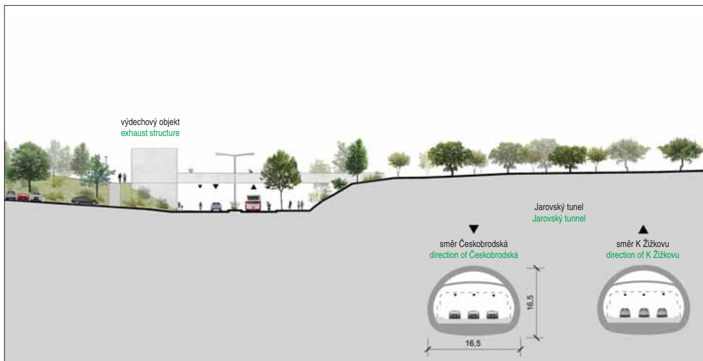
Obr. 4 Příčný řez profilem ulice Spojovací s Jarovským tunelem pod vrchem Třešňovka Fig. 4 Cross-section through Spojovací Street with the Jarov tunnel under Třešňovka Hill
