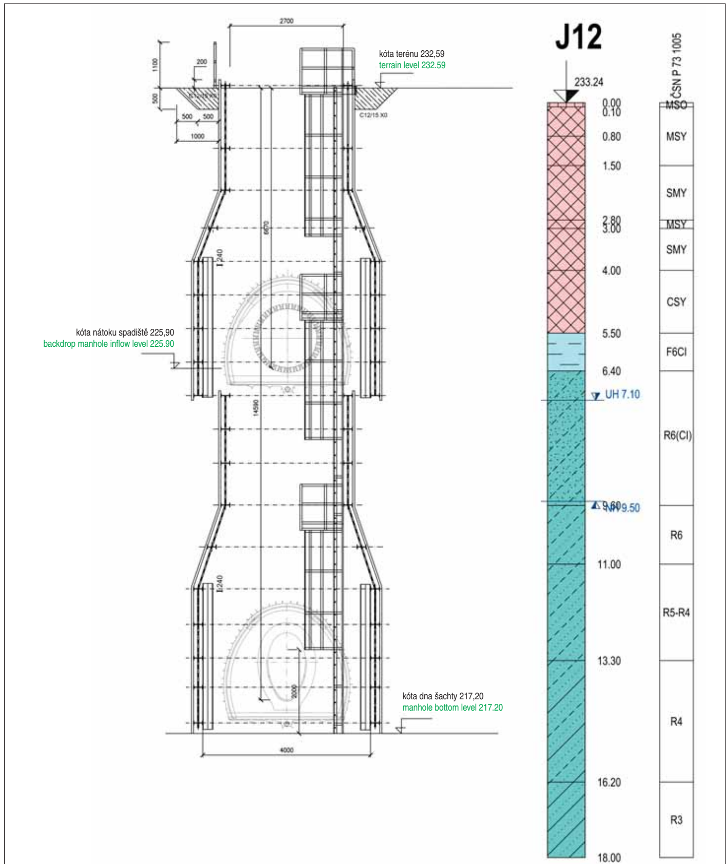
Obr. 7 Řez těžní šachtou TŠ9 (spadiště)
