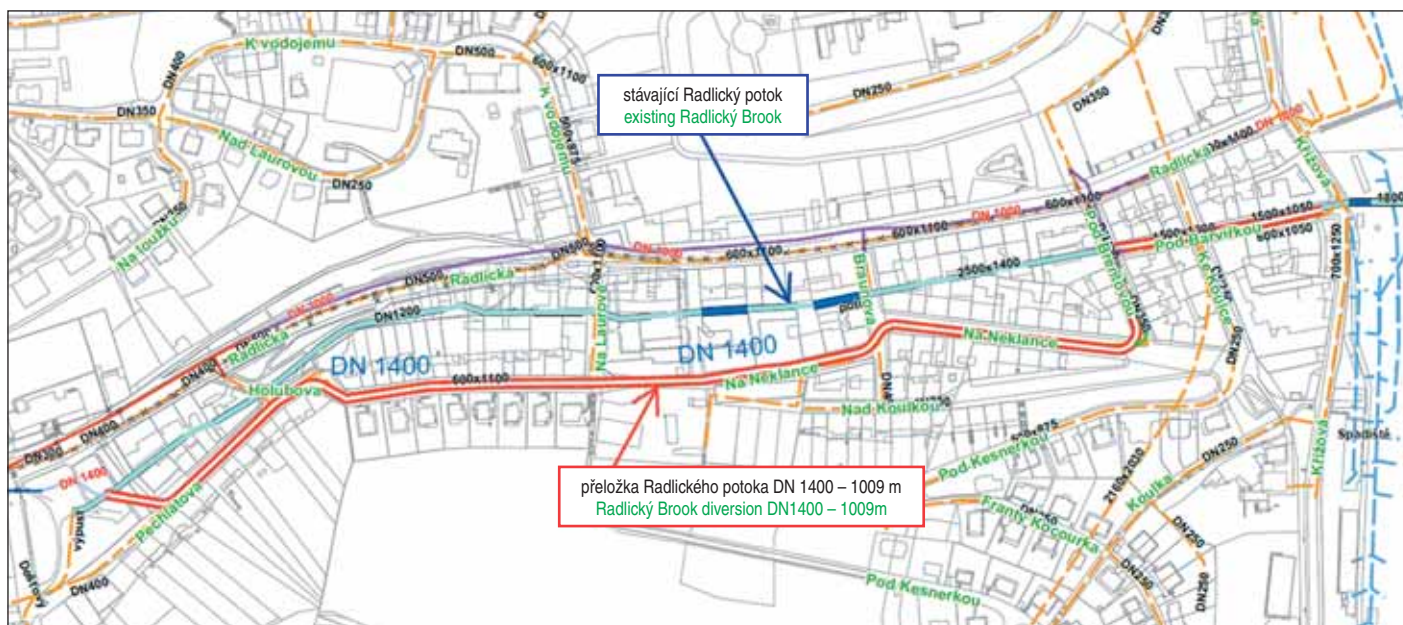
Obr. 3 Zákres navržené trasy přeložky Radlického potoka a stávajícího potoka ze studie
