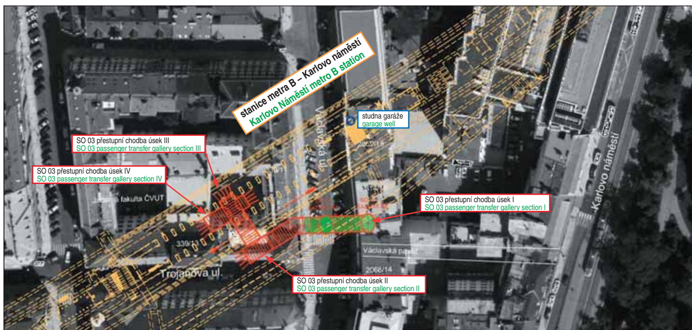
Obr. 1 Situace bezbariérového zpřístupnění stanice metra Karlovo náměstí s vyznačeným stavem ražeb k 12/2019 – na obr. zeleně vyšrafováno Fig. 1 Layout of step-free access to Karlovo Náměstí metro station in the state of excavation as of December 2019 – hedged green in the picture
