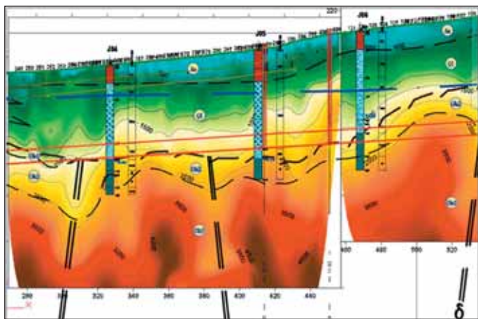
Obr. 4 Podélný geofyzikální profil – deprese ve skalních horninách zastižená v počátku měřeného úseku v rozmezí staničení 270÷500 m
