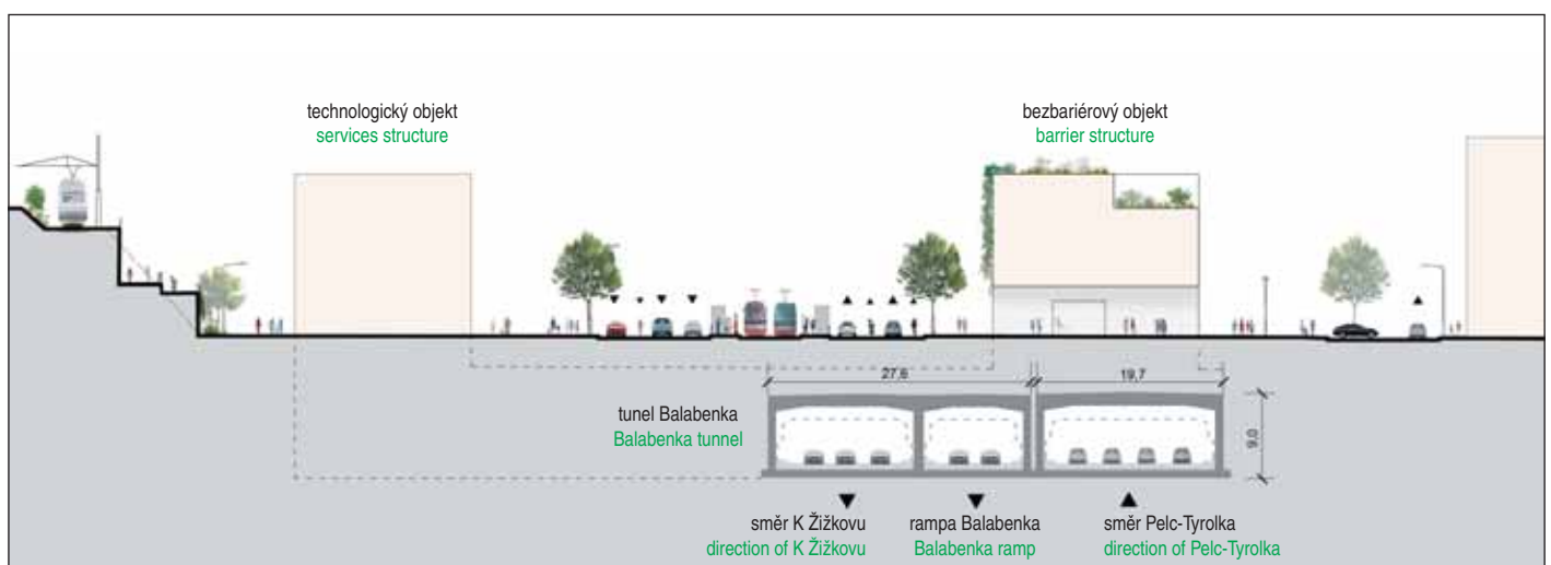
Obr. 3 Příčný řez v prostoru Balabenky Fig. 3 Cross-section in the area of Balabenka
