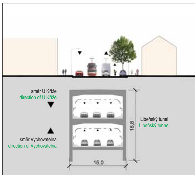
Obr. 6 Příčný řez Libeňským tunelem s patrovým uspořádáním v ulici Zenklova
