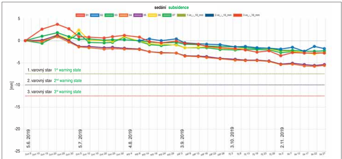
Obr. 9 Časový vývoj sedání bodů v profilu 2 v ul. Václavská – profil příčný na ražbu přestupní chodby – úsek II (výstup z informačního systému SIISEL) Fig. 9 Time development of subsidence of points in profile No. 2 in Václavská Street – profile transverse to excavation of the interchange gallery – section II (output from SIISEL information system)
