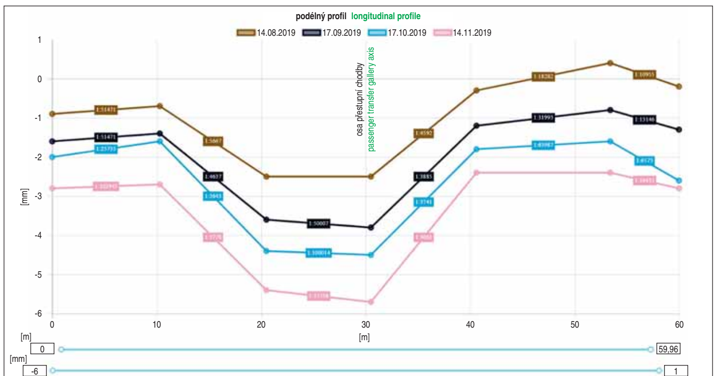
Obr. 10 Vývoj poklesové kotliny v profilu 2 v ul. Václavská nad ražbou přestupní chodby – úsek II (výstup z informačního systému SIISEL) Fig. 10 Development of settlement trough in profile 2 in Václavská Street above the excavation of the interchange gallery – section II (output from SIISEL information system)
