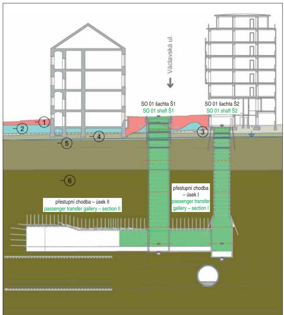
Obr. 3 Zjednodušený inženýrskogeologický řez s vyznačeným stavem ražeb k 12/2019: 1 – navázky; 2 – fluvialní sedimenty; 3 – břidlice silně zvětřalé; 4 – břidlice mírně zvětřalé; 5 – břidlice navětřalé; 6 – břidlice zdravé; modrá čára – průběh hladiny podzemní vody; červená čára – konvergenční profily v šachtách; světle zeleně vyšrafovaný stav hloubení a ražeb
