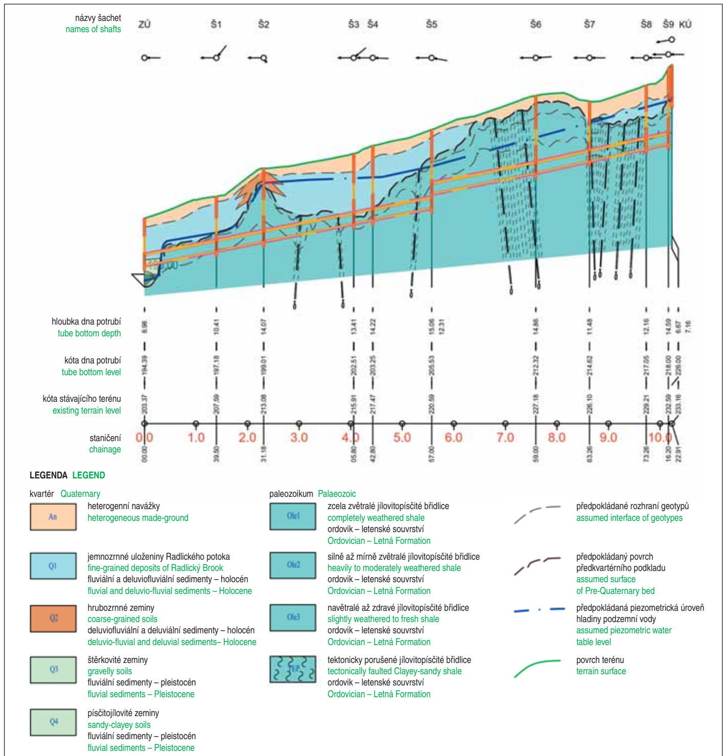
Obr. 5 Podélný geologický profil se zázřesem výsledků podrobného inženýrskogeologického a geotechnického průzkumu Fig. 5 Longitudinal section with results of the detailed engineering geological survey and geotechnical investigation drawn in it
