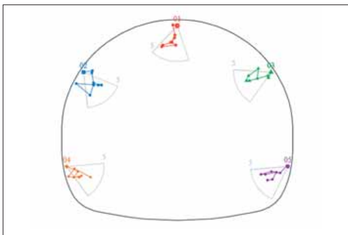
Obr. 6 Vektorový diagram polohových změn konvergenčních bodů profilu v přestupní chodbě
