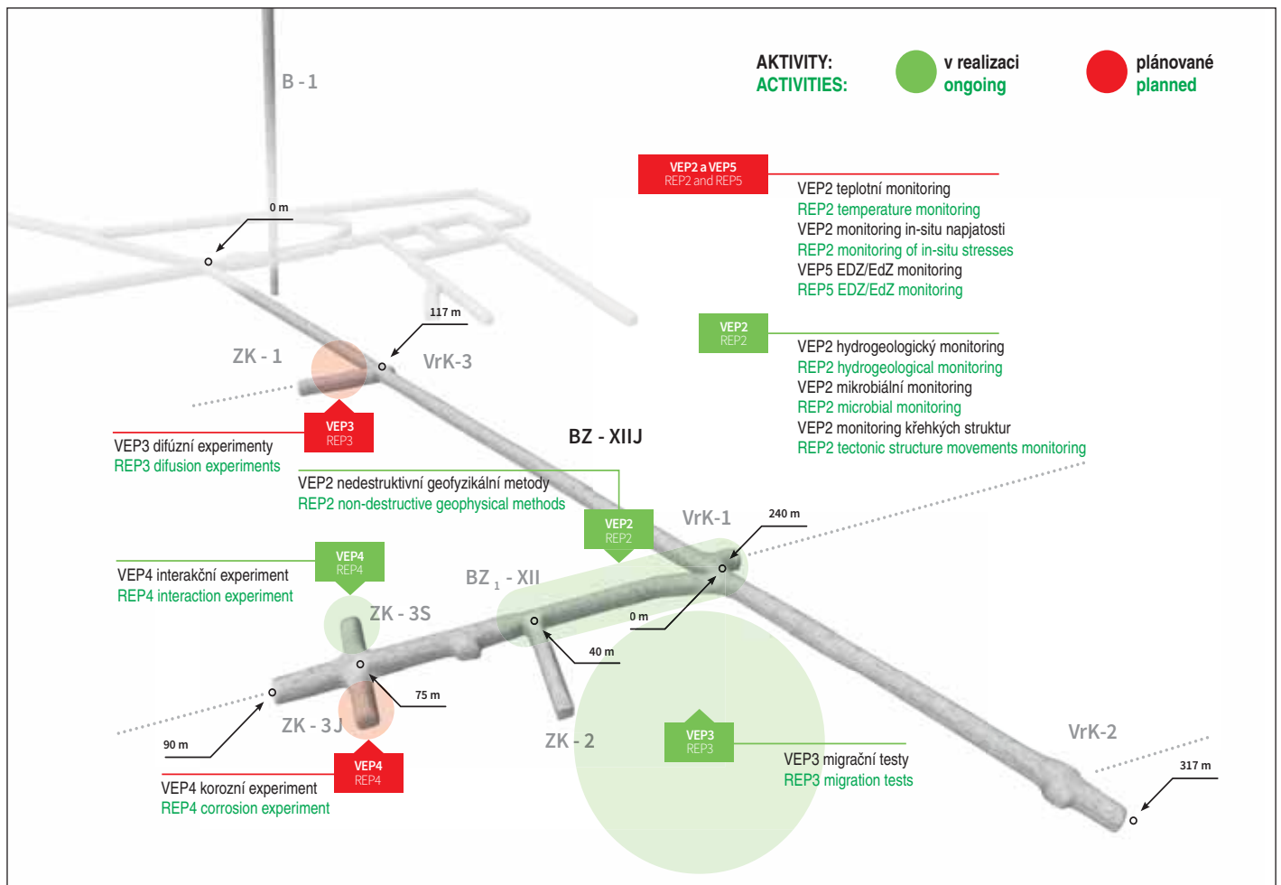
Obr. 3 Prostorové schéma PVP Bukov s vyznačením probíhajících a plánovaných aktivit Fig. 3 Spatial scheme of the Bukov URF indicating ongoing and planned research activities
